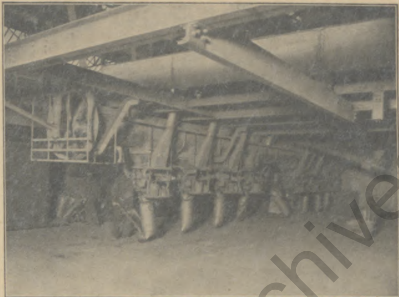
Abfäderei mit acht automatischen Füll- und Wiegestellen.
