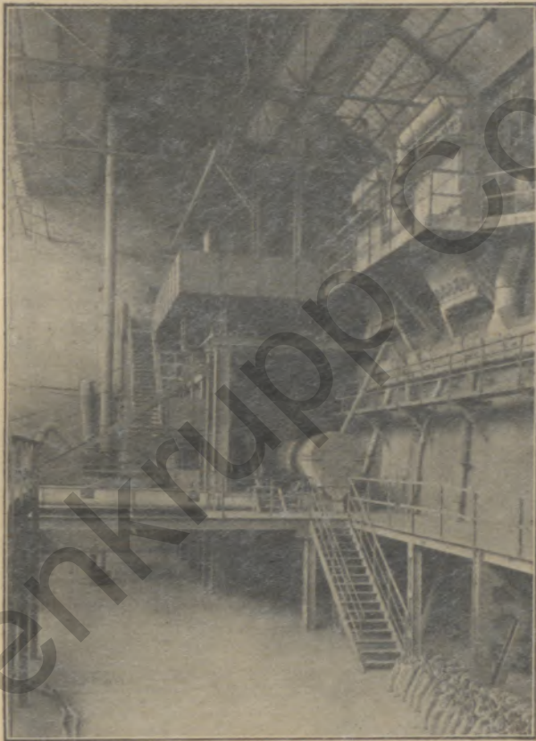
Gesamtansicht der Mühlengruppe II mit Entstaubungsanlage.
