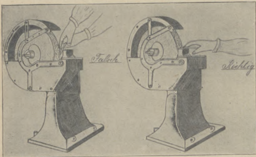
Falsche und richtige Stellung der Schleifvorlage an Schmirgelsteinen. Zeichnung von Betriebsführer a. D. Perker.
