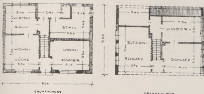
EINZELHAUS
