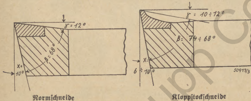
Normschneide
