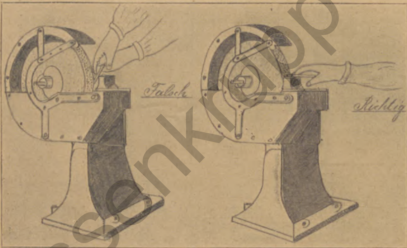
Falsche und richtige Stellung der Schleifvorlage an Schmirgelscheiben.
