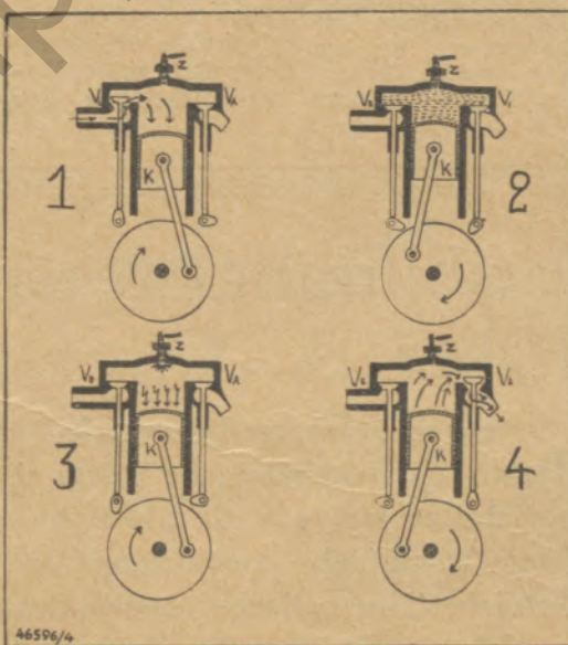
Abb. 2: Schematische Erläuterung der Arbeitsweise des Viertaktmotors
