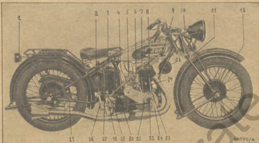
Abb. 1: „Ardie“, 500 ccm, untergesteuert, 14 PS bei 3900 Umdrehungen i. d. M.
