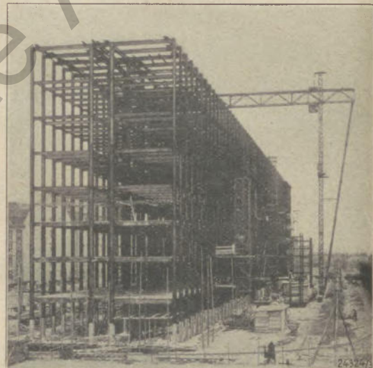
Stahlstelet des Siemens-Hochhauses in Berlin, erbaut von der Brückenbauanstalt der Dortmunder Union
