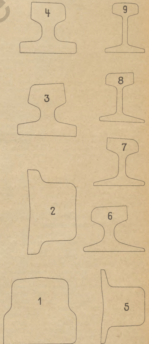
Stichfolge einer Eisenbahnschienen-Kalibrierung vom Block bis zum Fertigprofil
