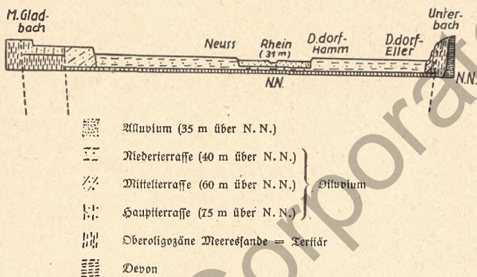
Abb. 3. Profil M.Gladbach — Unterbach (bei Düsseldorf)
