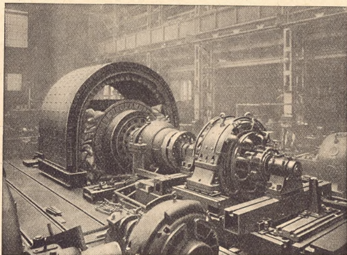
Abb. 7. Der Läufer im Versuchsfeld
