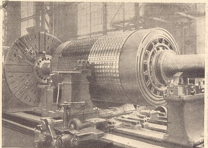
Abb. 5. Der Läufer auf der Drehbank
