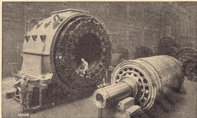
Abb. 9. Ständer und Läufer fertig gewickelt
