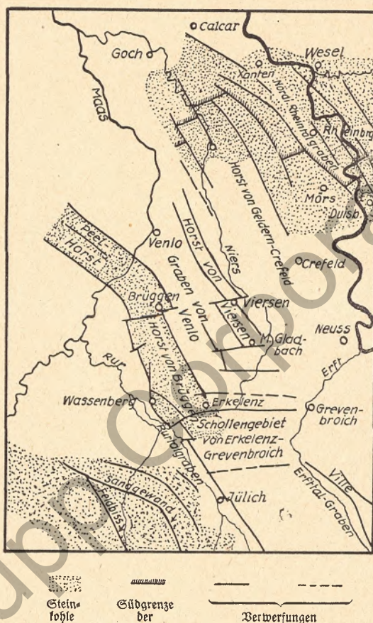
Abb. 1. Tektonische Skizze des Niederrheingebietes
