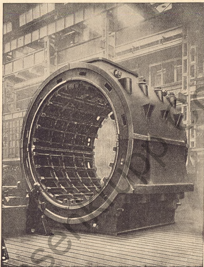
Abb. 8. Das Ständergehäuse
