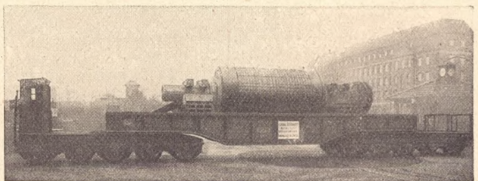
Abb. 6. Der fertige Läufer auf seinem Sonderwagen
