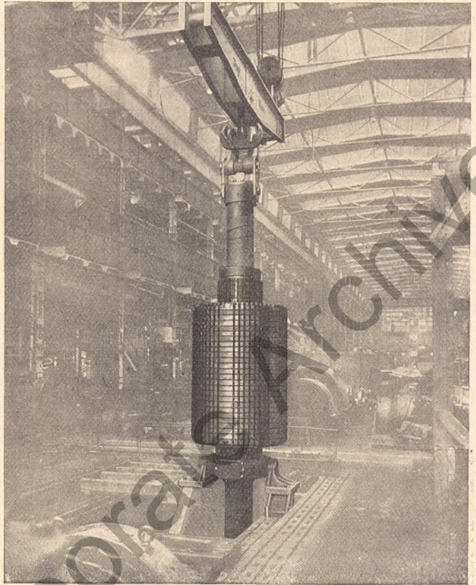
Abb. 4. Aufbringen der Läuferplatten auf der Läuferwelle
