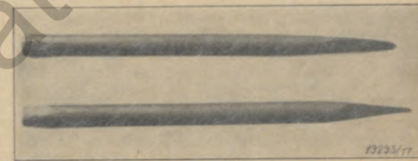
Bild 7: Facharbeit für Bauschlosser: Flachmeißel (schlechte und gute Ausführung)
