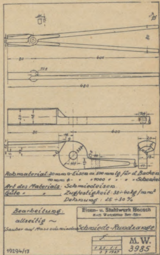
Bild 8: Facharbeit des Schmiedes: Schmiedes-Rundzange (Aufgabe)
