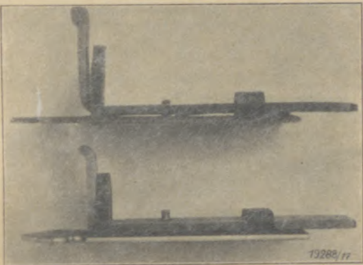
Bild 2: Facharbeit für Bauschlosser: Türriegel (schlechte und gute Ausführung)
