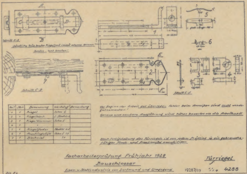
Bild 1: Facharbeit für Bauschlosser: Türriegel (Aufgabe)
