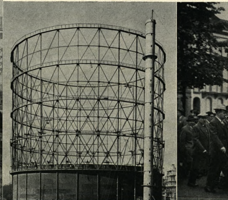
Einer der größten Glockengasbehälter (200 000 cbm Speicherraum) mit geschweißten Hubteilen wird bei den Chemischen Werken Hüls von der Firma Klönne gebaut. Wir lieferten 880 t Stahl, die August Thyssen-Hütte 490 t
