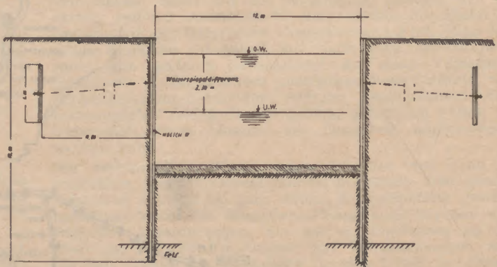
b. Ausführung mit Stahlpundwänden
