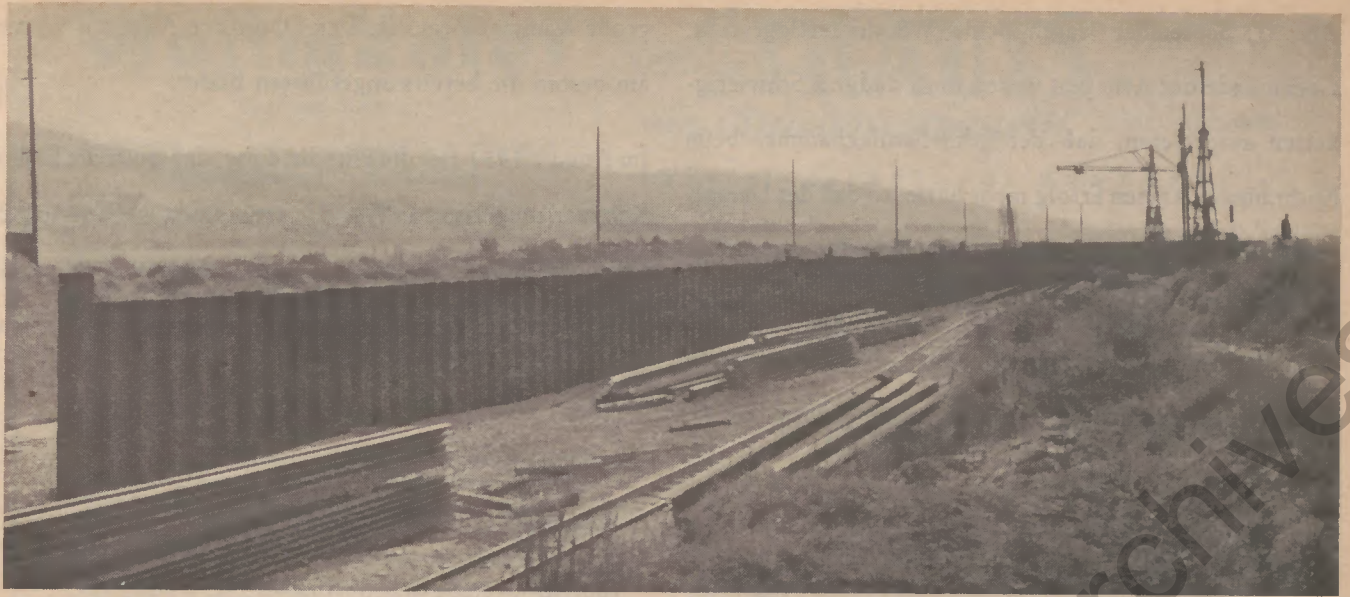
Bild 12: Flußseitige Kammerwand
