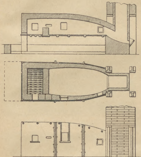
Abb. 9: Buddelofen mit Eisenherd und Gießplattenmantel
