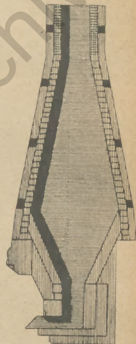
Abb. 10: Erster Kokshochofen in Gleiwitz (1794)
