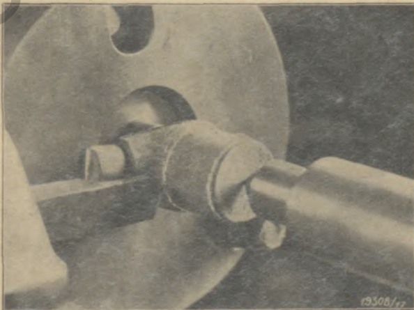
Bild 16: Facharbeit für Dreher: Anreihen der radialen Zapfenmitte und der Anlagabstände mit dem Drehstuhl
