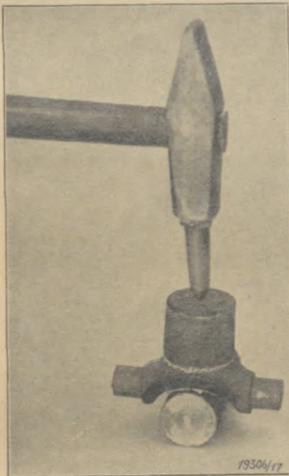
Bild 14: Facharbeit für Dreher: Richtiges Anfröhen
