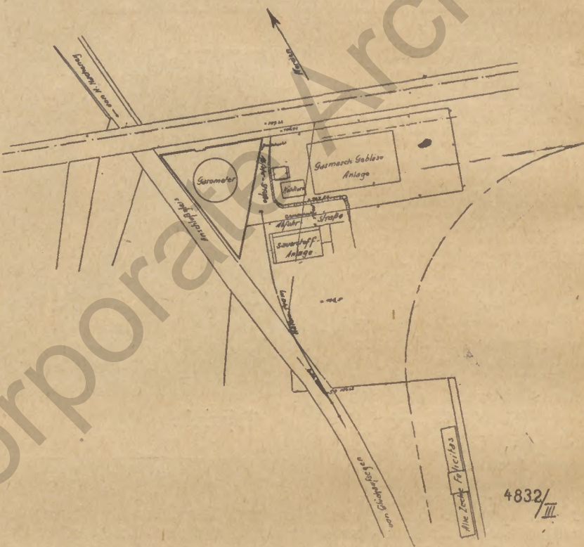
Lageplan zum Bau einer Sauerstoffanlage mit Gleisanlage
