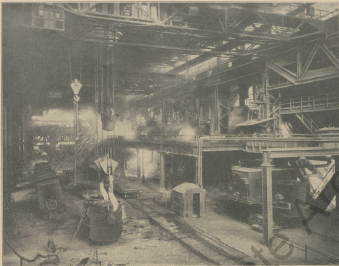
Thomaswerk
