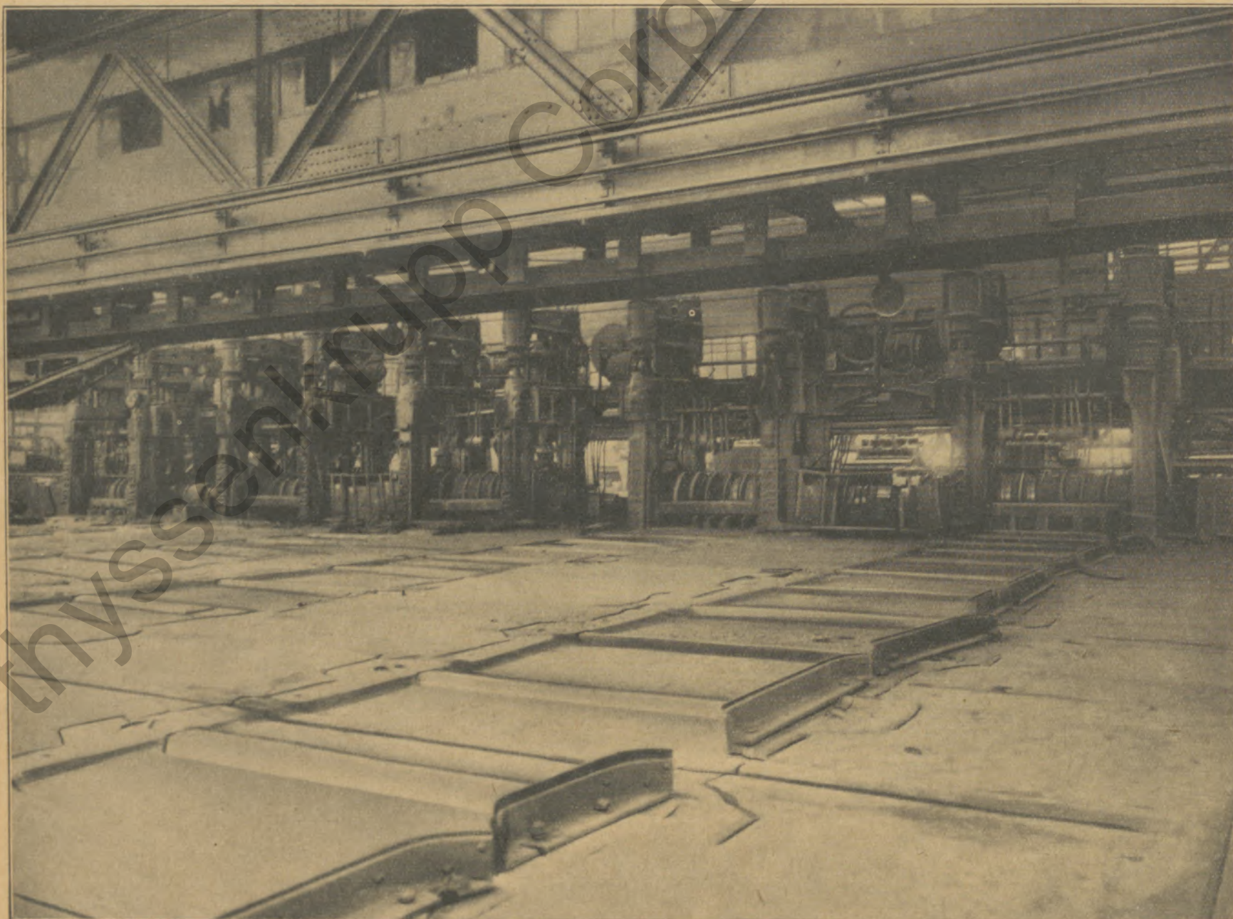
Fertigstraße I
