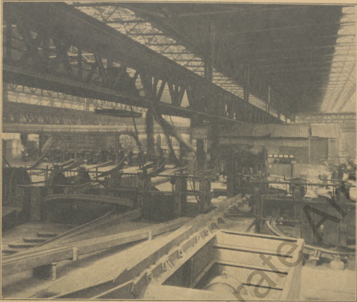
Drahtstraße
