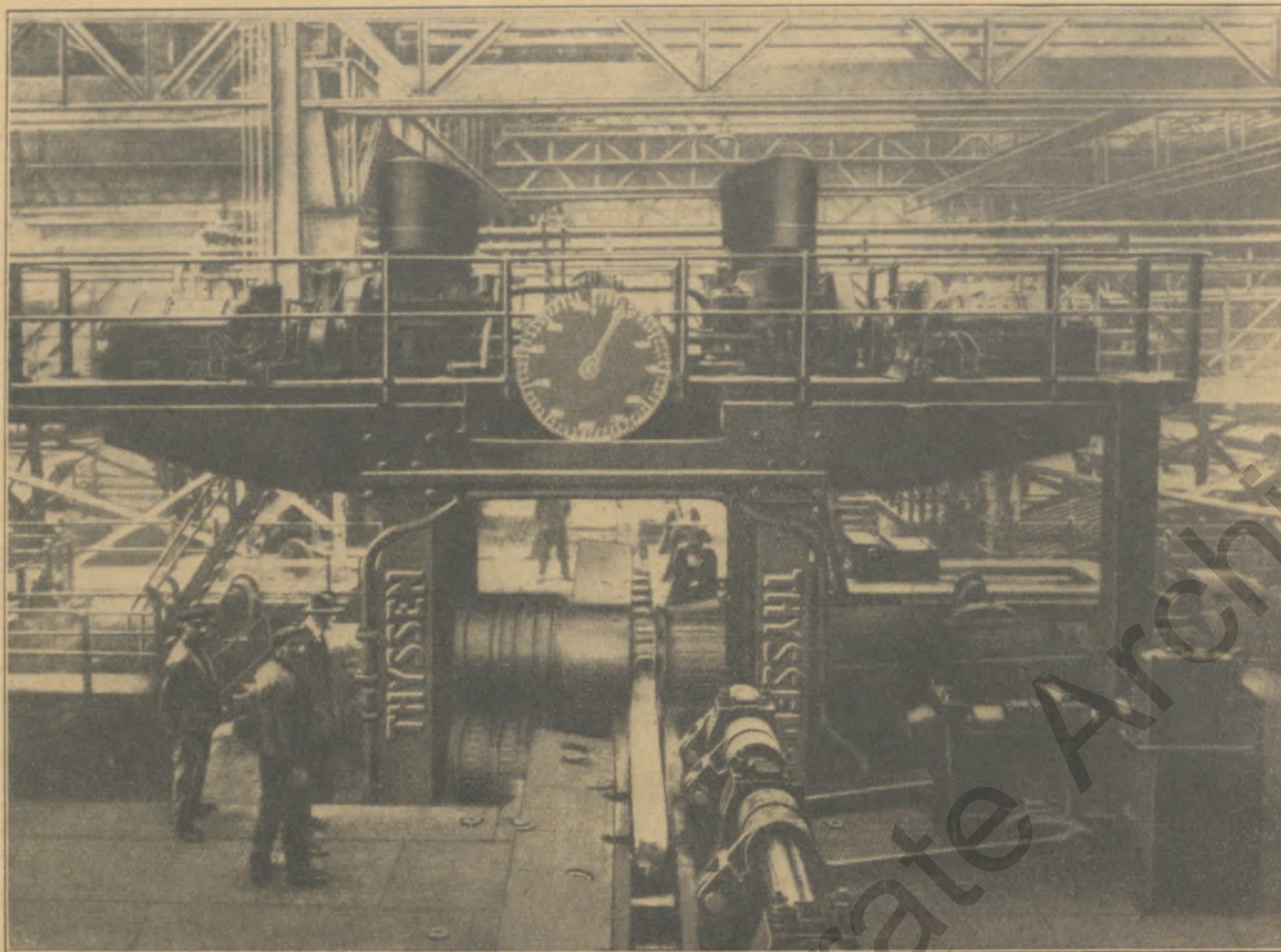
Blockstraße III
