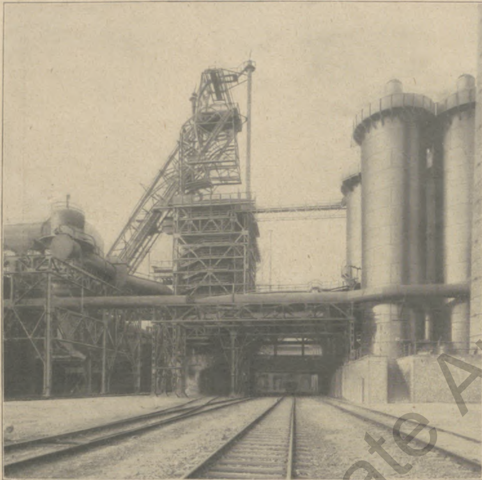
Hochofen VIII
