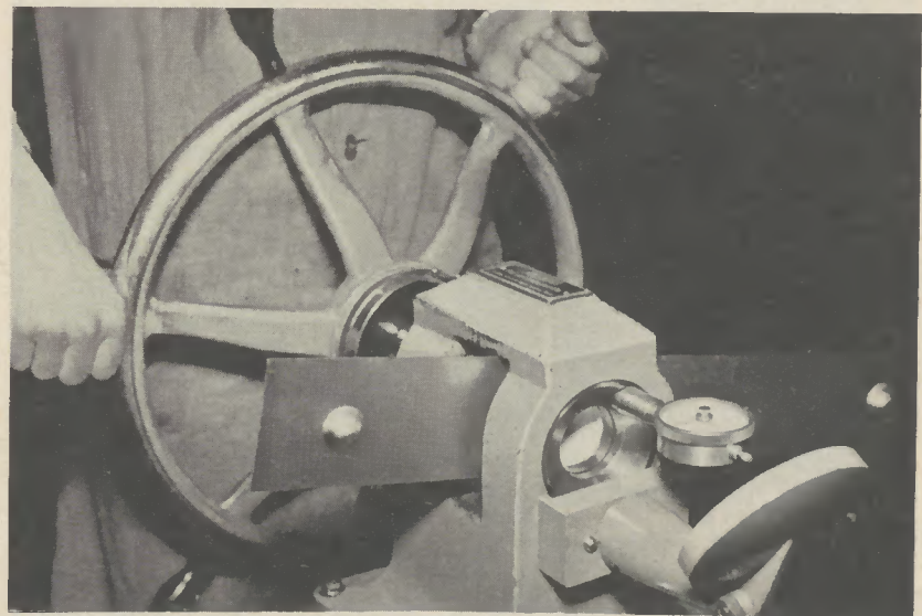
Tiefungsdrücken mit der Hand nach „Erichsen“
