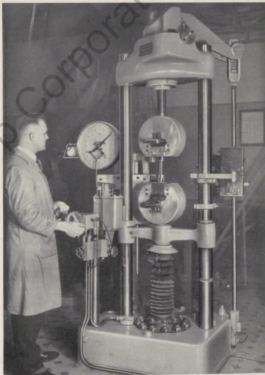
Auf der Zerreißmaschine werden die Festigkeiten des Stahles geprüft
