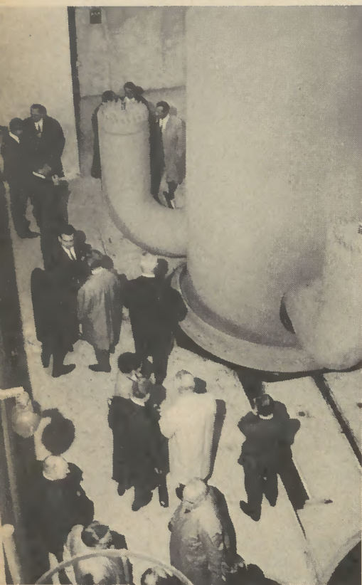
In der sieben Meter tiefen Montagegrube betrachten die Besucher den mächtig aufragenden Druckbehälter
