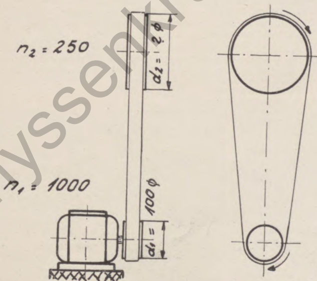
Offener Riemen
