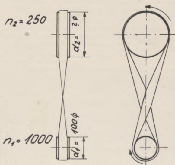
Gekreuzter Riemen
