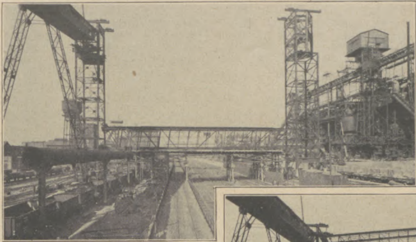
Brücke auf einem Gerüst über der Köln-Mindener Bahnstrecke ruhend
