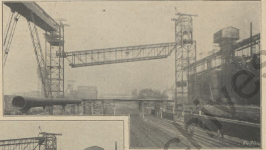
Brücke während des Hochziehens
