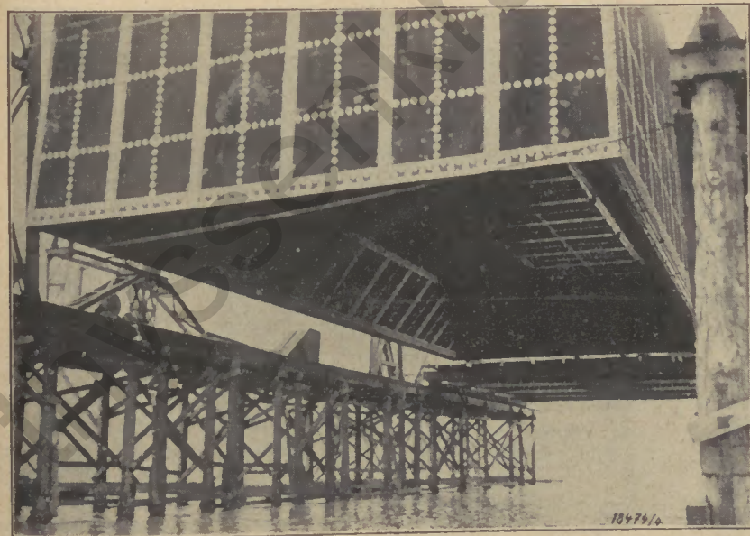
Schneiden und künftige Arbeitskammer des in den Absenkböcken hängenden Caissons
