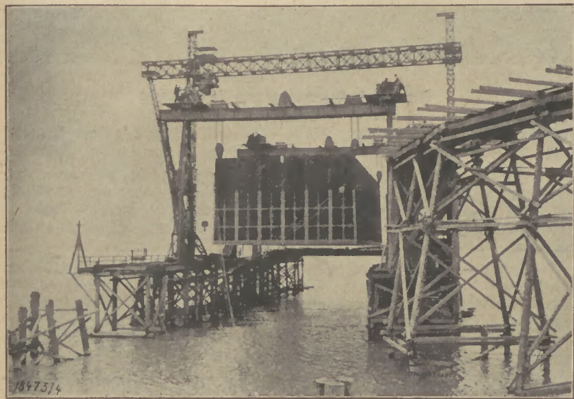
Das Zuwasserlassen des ersten Caissons Anfang Mai 1928
