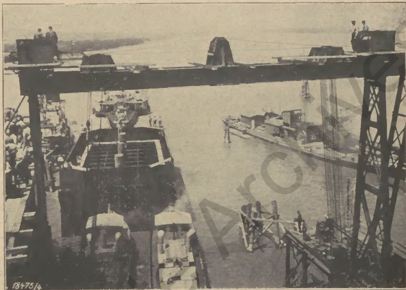
Das Abschleppen des ersten Caissons zur Verwendungsstelle
