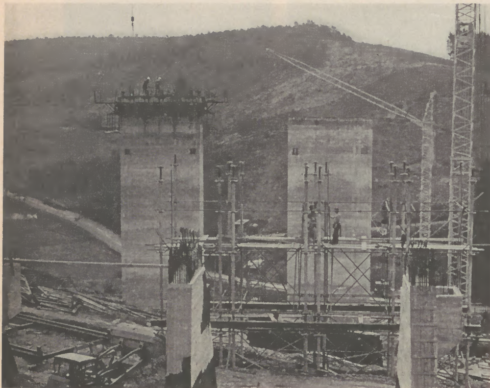
Bundes-Autobahn-Talbrücke bei Eisern
