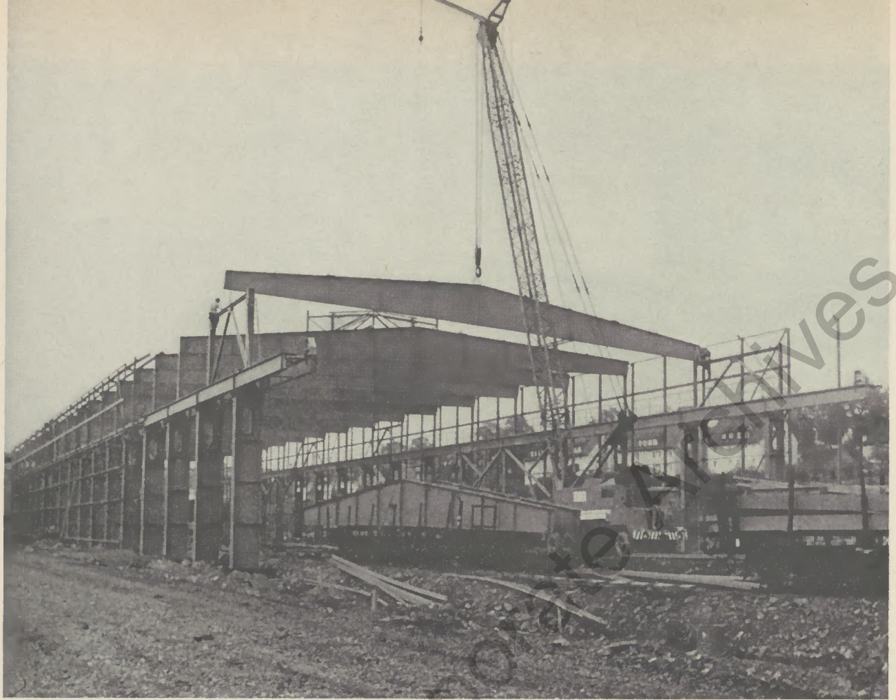
Stahlkonstruktion für die neue Bandverzinkungs- anlage im Werk Eichen. Die Aufnahme entstand vier Wochen nach Montagebeginn. Sie zeigt den niedrigen Hallenteil vor der Errichtung der hohen Rahmenkonstruktion. Montage der vollwandigen Dachbinder, die mittels Autokran direkt vom Waggon abgenommen und auf die eingespannten Stützen aufgesetzt werden.
