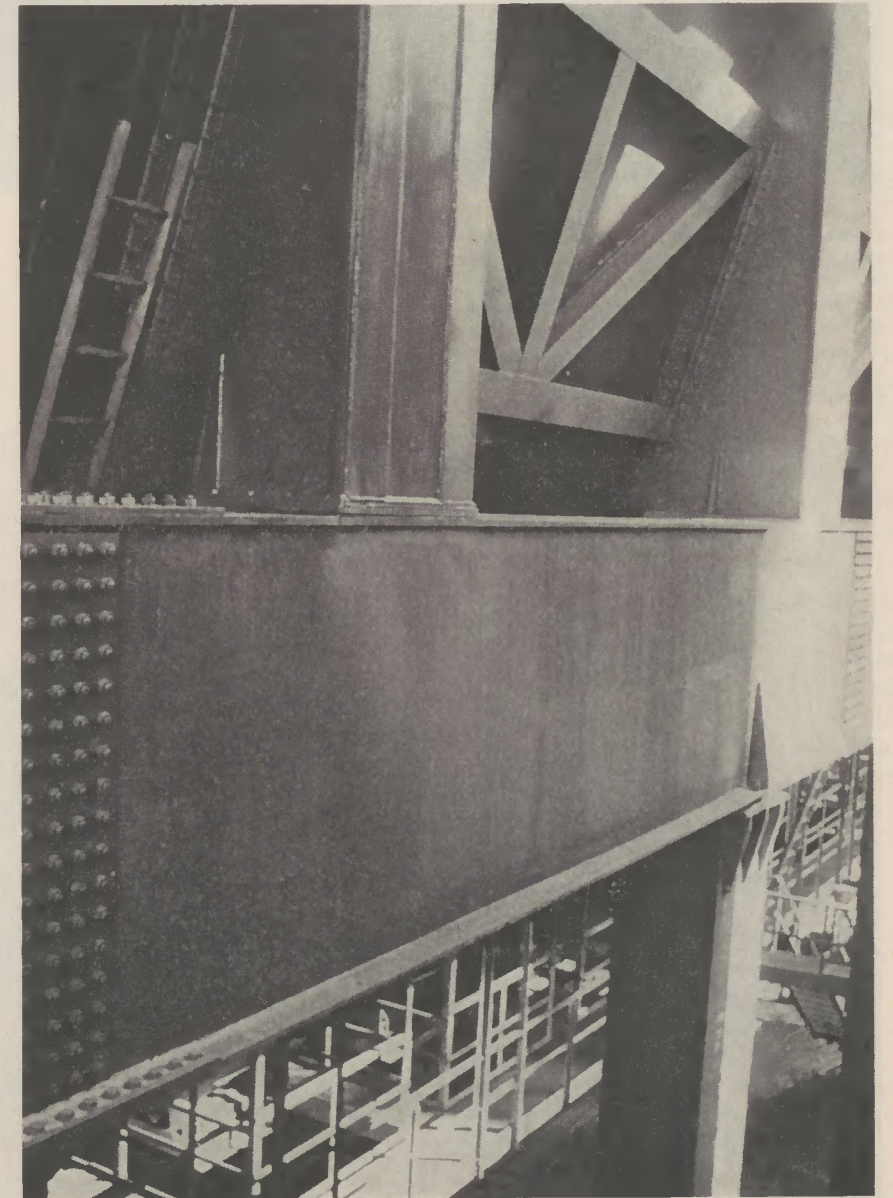
Schwere, geschweißte Stahlkonstruktion für eine Erz- und Koksunkeranlage im Ruhrgebiet. Die Anlage hat eine Höhe von ca. 15 m. Die Bauteile hatten Stückgewichte bis zu 20 t. Einige Montageverbindungen erfolgten mittels hochfester Schrauben.
