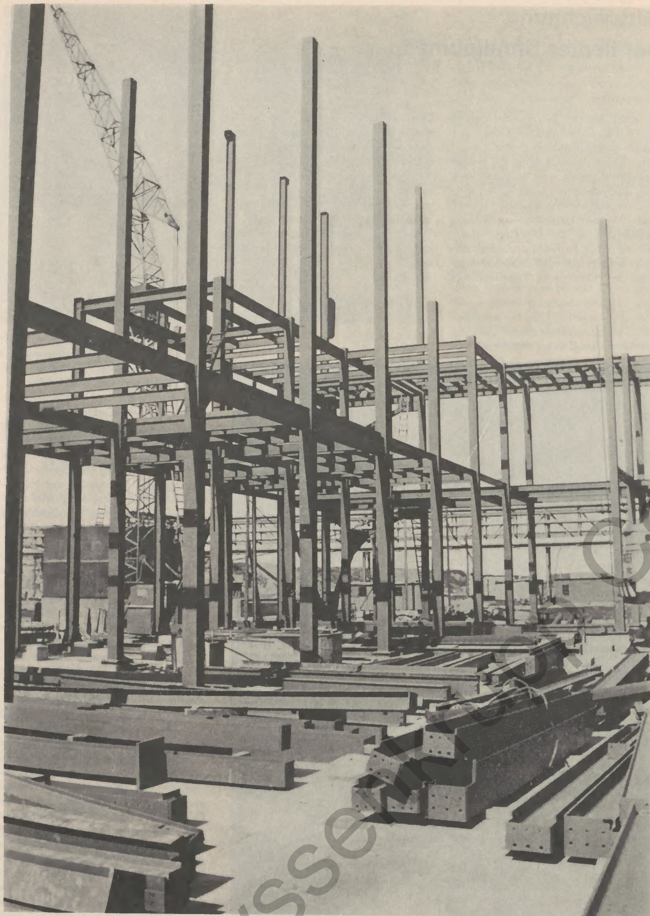
Stahlkonstruktion für ein mehrgeschossiges Fabrikationsgebäude der chemischen Industrie
