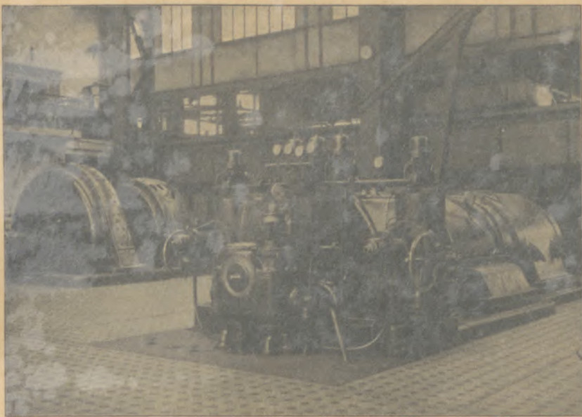
Abb. 30: Mitteldruck-Kondensations-Turbosatz, gebaut 1924 von Brown, Boveri & Cie., Mannheim. Leistung: 5700 Kilowatt, minütl. Drehzahl: 3000, Frischdampfdruck: 12 at
