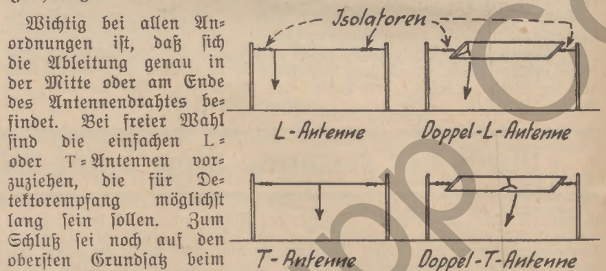
Abb. 3: Antennenformen.
