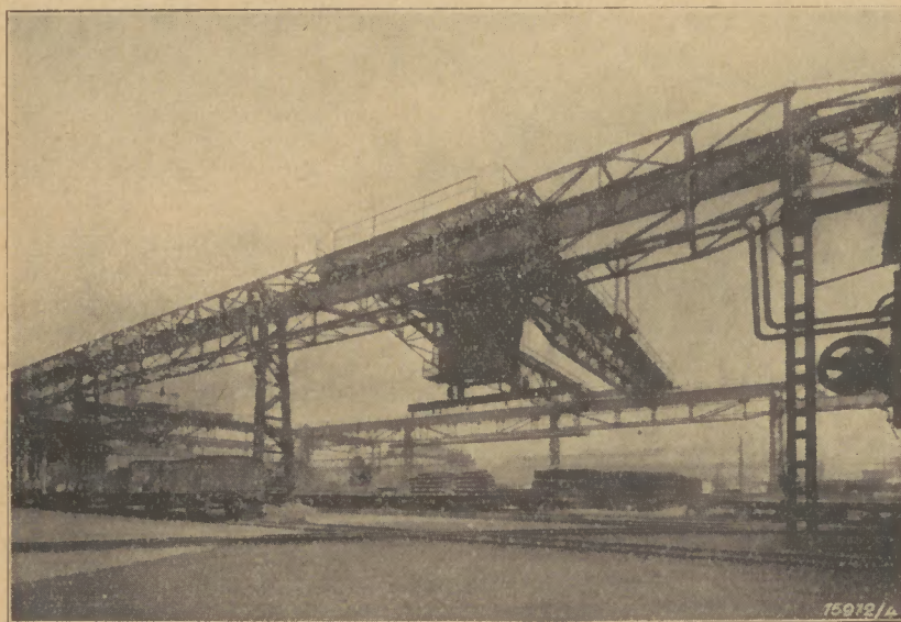
Abb. 5: Neuer Kranbahnenteil mit 10 t Kran
