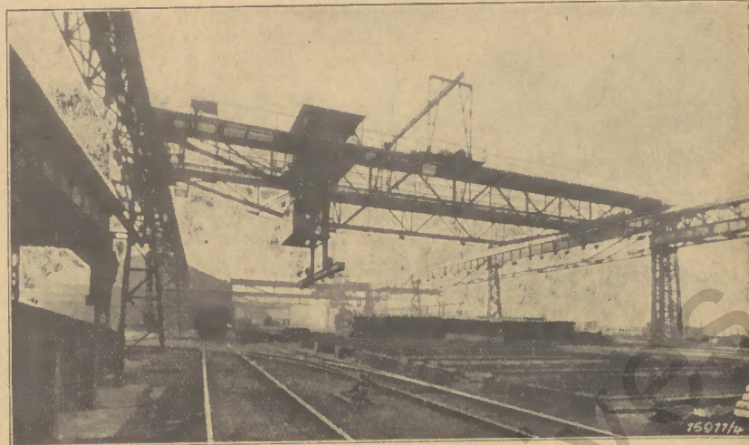
Abb. 4: Neuer Teil der Längsfranhahn mit 10 t Kran
