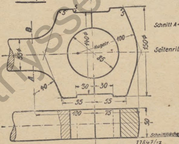
Ausgangsaufgabe f. Maschinenschlosser: Schubstangenkopf
