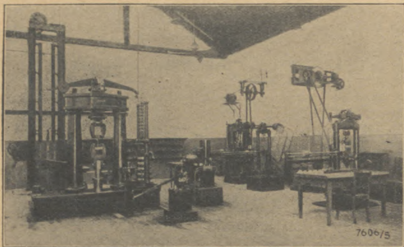
Prüfungsraum mit Zugversuchsmaschinen
