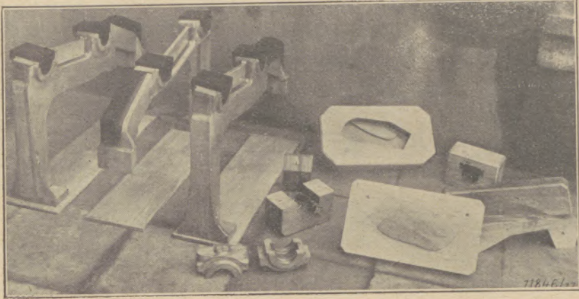
Abb. 4: Einheitsstück der Modelltischler-Lehrlinge
