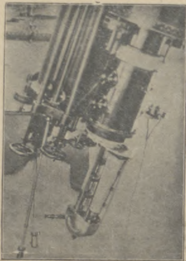
Spektrograph am großen Fernrohr des Potsdamer Observatoriums, mit dem die Spekttralaufnahmen gemacht werden, die uns genaue Aufschlüsse über die physikalische Beschaffenheit ferner Himmels- körper geben.
