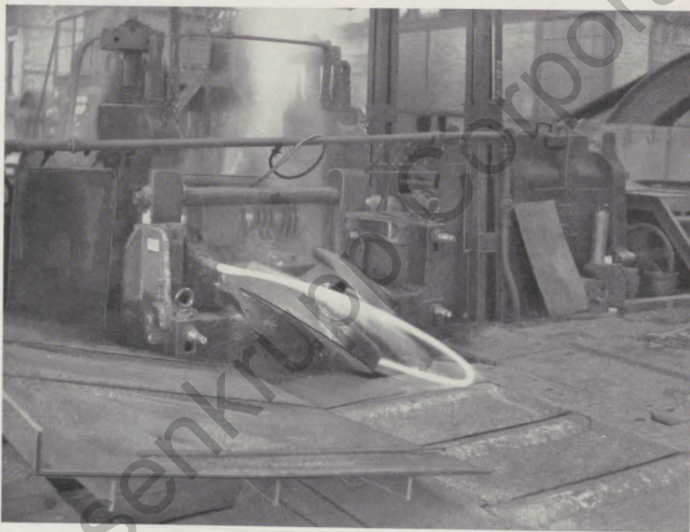
Bild 4: Neue selbsttätige Umföhrung an der Vorstraße der Feinstraße in Willich
