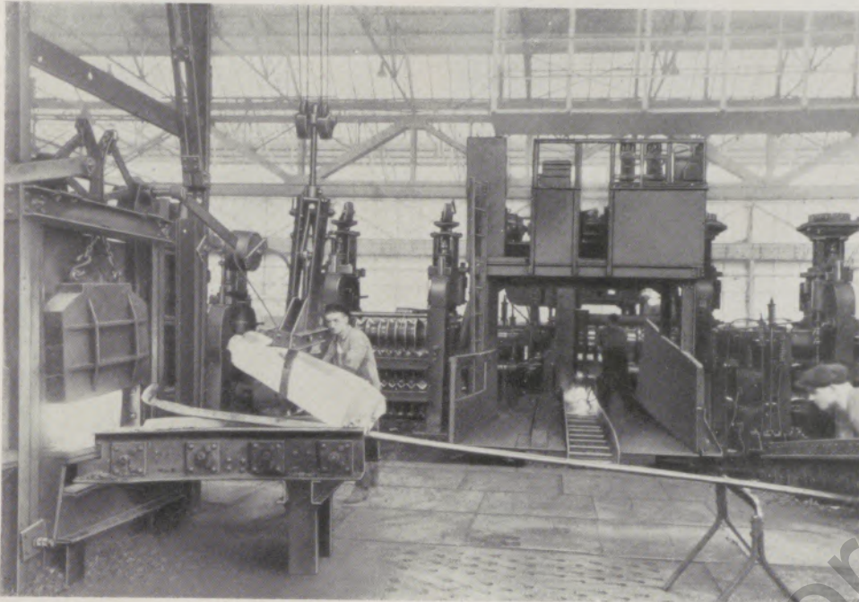
Bild 1: Teilansicht unserer Blockstraße in Krefeld
