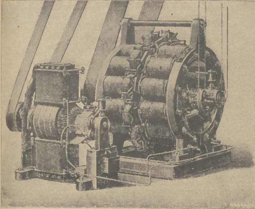
Wechselstrom-Maschine von Siemens & Halske mit dynamo-elektrischem Stromerzeuger
