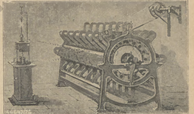
Magnetoelektrische Maschine
