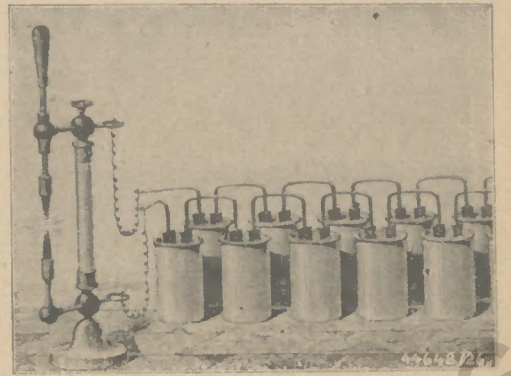
Davy'scher Lichtbogen, erzeugt durch galvanische Säule
