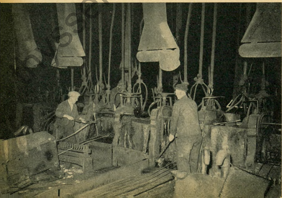
Am schnellsten muß das Fassen und Einstecken gehen, wenn 5 mm gewalzt wird und Draht rotglühend an Draht läuft
