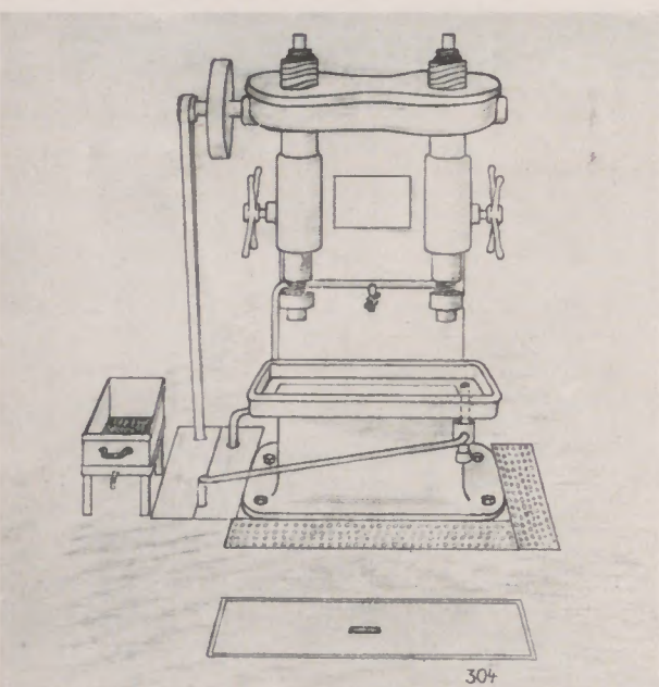
Skizze der Maschine nach der Umgestaltung
