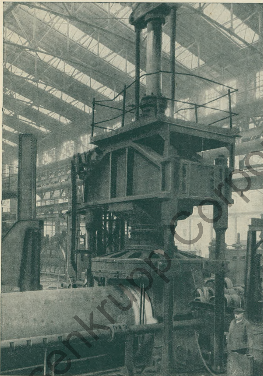
Zusammenbau des Trommelsendes einer Hochsicherheitstrommel unter der hydraulischen Presse.
