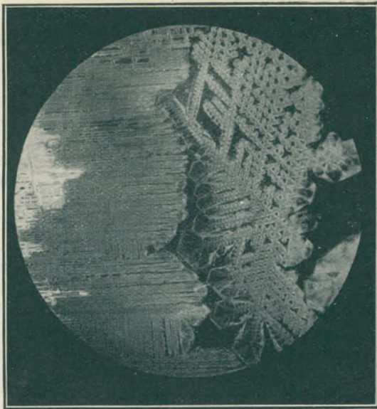
Abb. 1. Kristallskelett.
