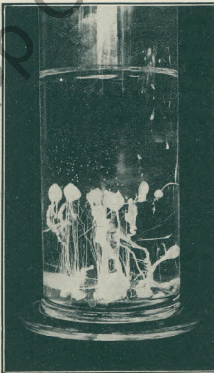
Abb. 3. Silikatblüten. (Nickelchlorid und Mangansulfat.)
