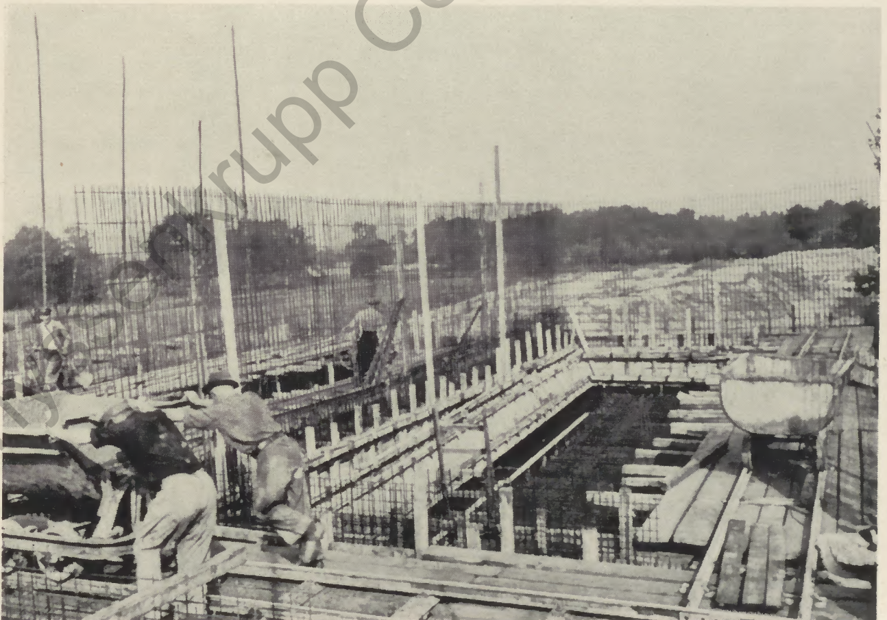
Baustahlgewebe bei der Bewehrung von Wasserbecken
