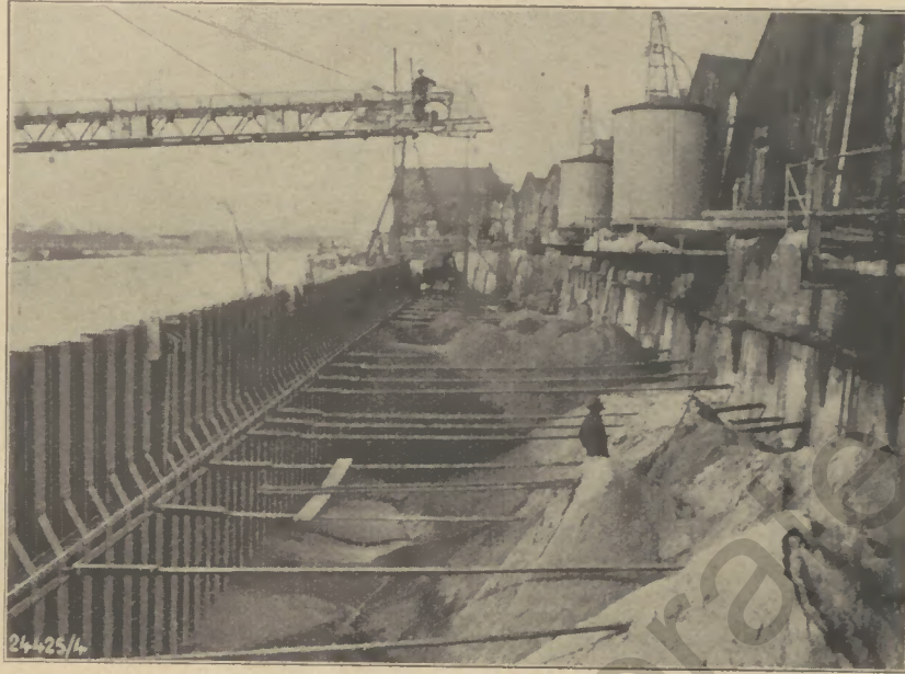
Kaimauer aus Spundwandeneisen „Larssen“ der Dortmunder Union beim Umbau des Weserbahnhofes in Bremerhaven
