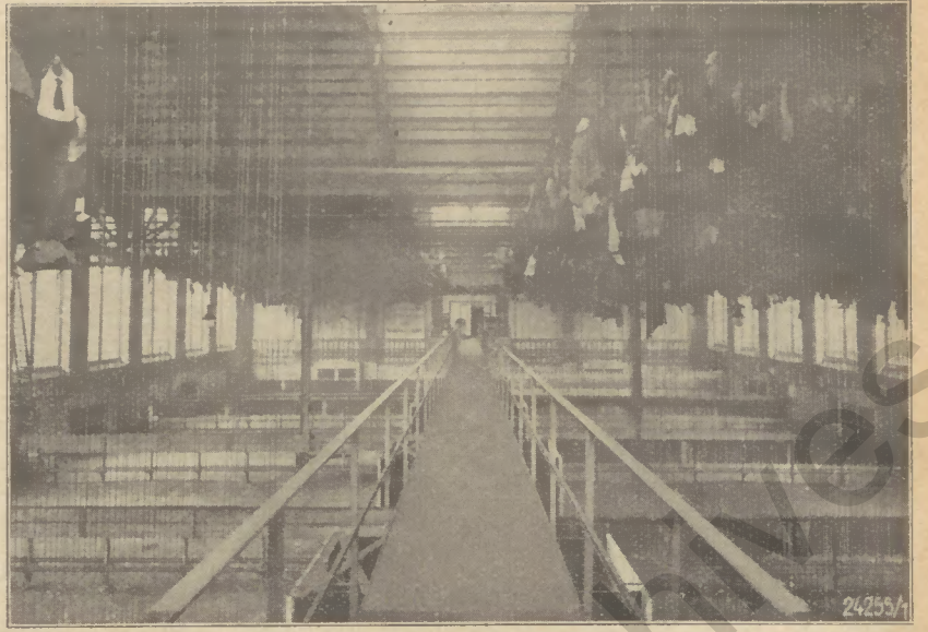
Waschklaue einer Zeche
