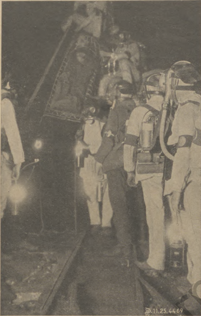
Verletzten-Transport mit Sarczyks Steiltransportbahre des Draeger-Werks, Lübeck.
