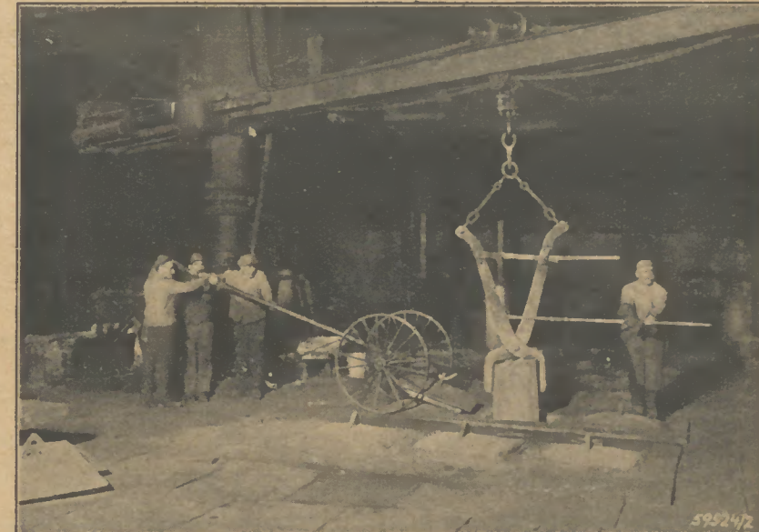
Alter hydraulischer Grubentran und Bedelstarre — Tiefofenanlage Walzwerk III
