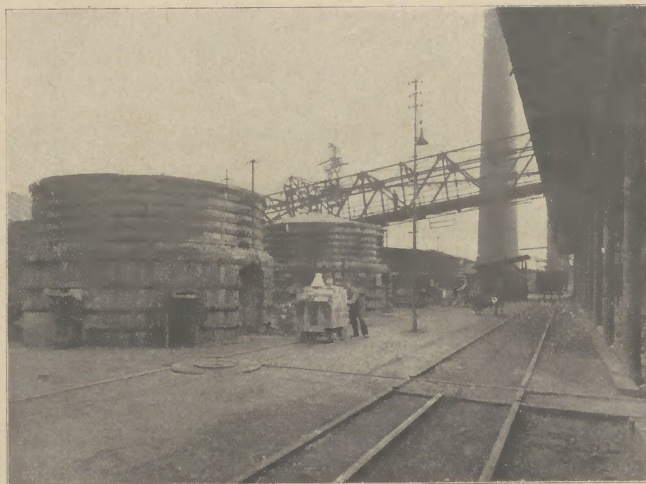
Steinbrennofen, im Vordergrund ein Wagen mit gebrannten Steinen, die zum Lager gefahren werden
