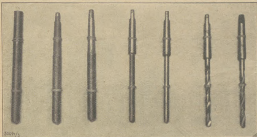
Abbildung 2: Werdegang des gefrästen Bohrsers
