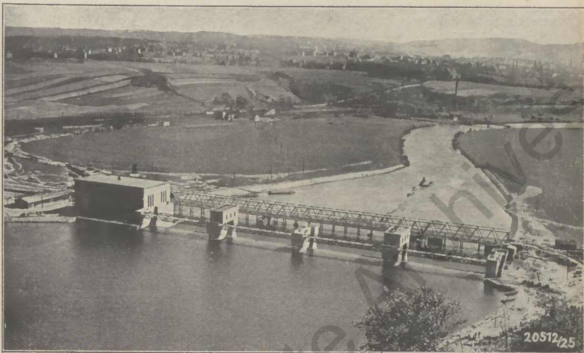
Bild 1: Wehranlage in der Ruhr bei Hengstey. 2 Versenkwalzen, 1,8 m absenkbar, und 2 normale Walzen, je 30 m Lichtweite, 6 m Stauhöhe
