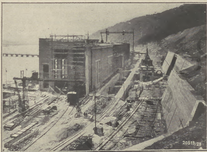
Bild 2: Pumpspeicherkraftwerk Herdecke im Bau
