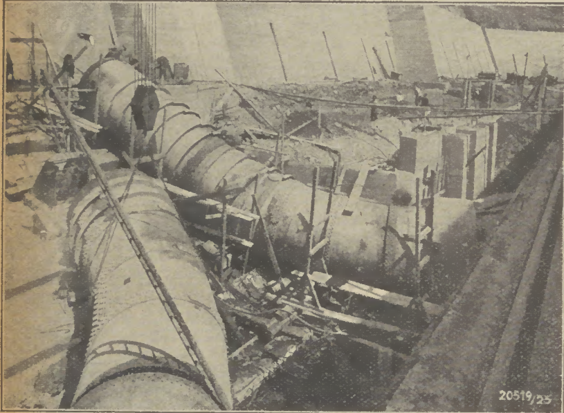
Bild 8: Die Rohrleitung beim Zusammenbau
