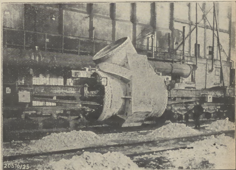
Bild 5: Ein „gewichtiges“ Stück auf dem Transport. Rohrteilungsstück vor dem Krafthaus, 35 000 kg Gewicht, auf einem Tiefladewagen
