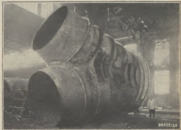
Bild 4: Hofenrohr zur Teilung der Leitung in 2 Stränge am Austritt des Stollens. Durchmesser 5 m und 2 mal 3,20 m
