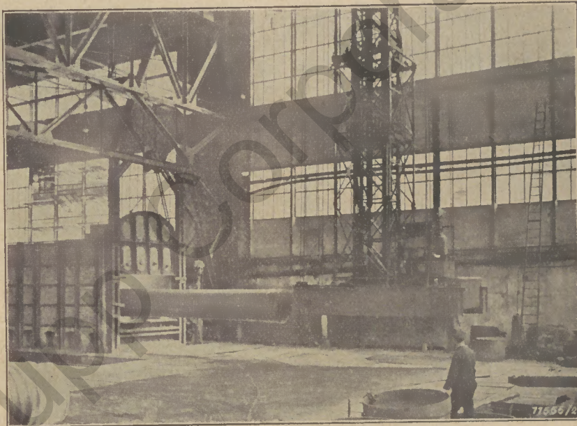
Abb. 3: Rohrglühofen; Einbringen eines fertig geschweißten Rohres mit dem Löffelkran
