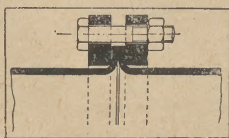
Fig. 8: Bördelst.-Verbindg.
