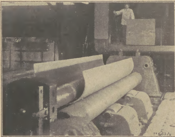
Abb. 1: Biegemaschine. Biegen eines Bleches
