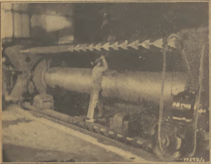
Abb. 4: Biegemaschine. Rundieren eines Rohres
