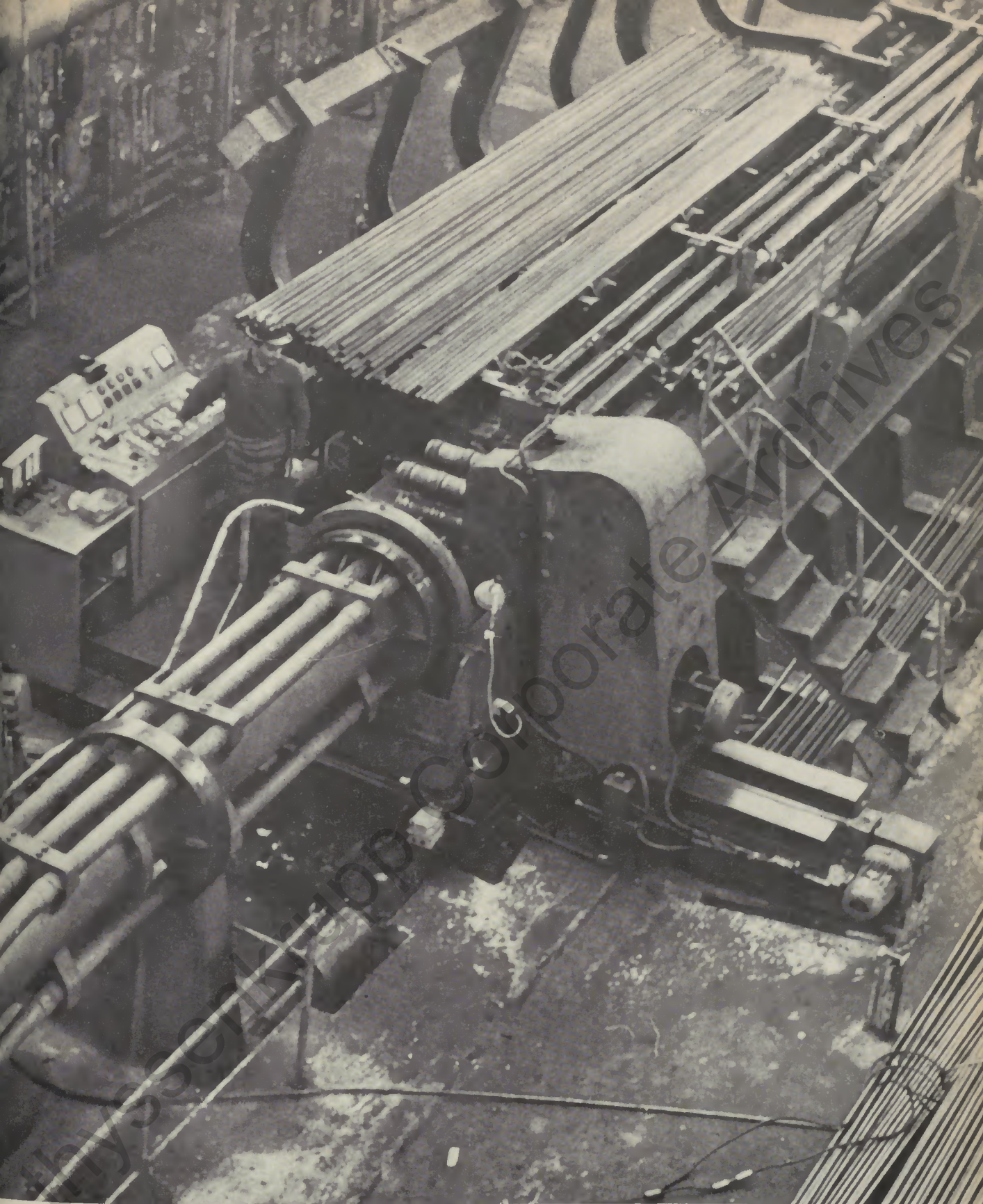
Eine halbautomatisch arbeitende Dreifach-Ziehbank.
