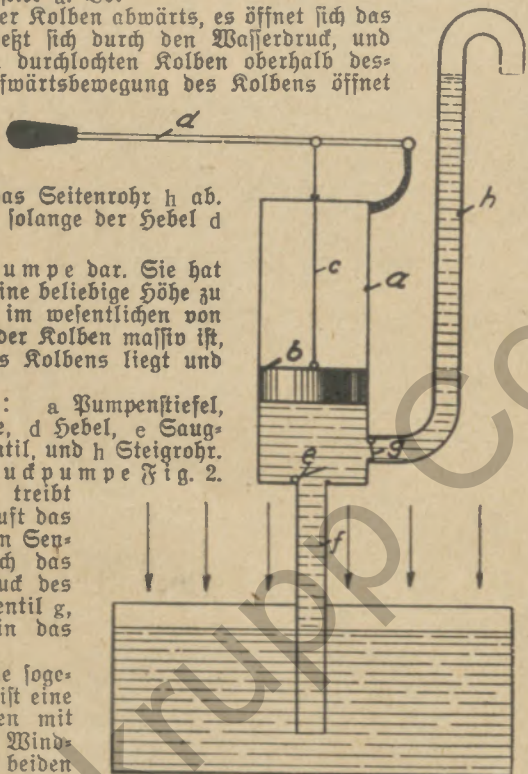
Fig. 2: Druckpumpe
