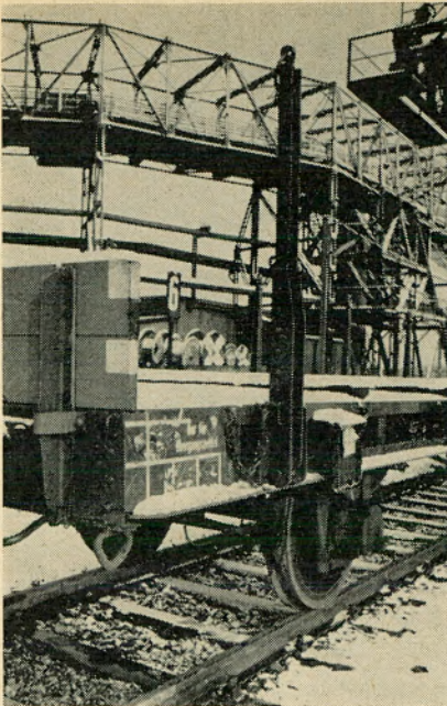
Vorstehendes Bild zeigt die Runge mit Sicherungsbolzen.
