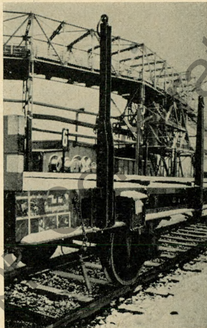
Auf diesem Bild ist der Bolzen herausgezogen. Vorsicht! Gefahr! Bolzen nach dem Hochstellen der Runge sofort einstecken. Sonst geht es wie
