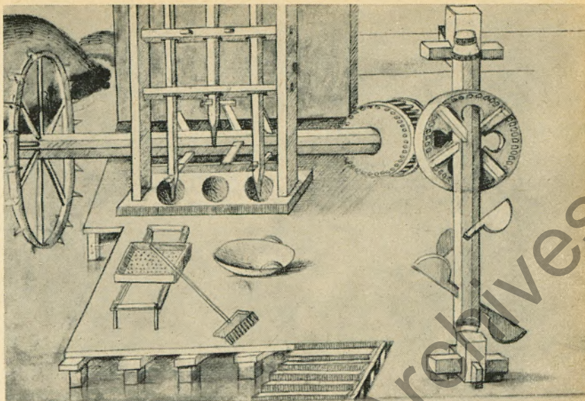
Abb. 2 Mittelalterliches Hausbuch um 1480, Stampfwerk für Mineralien
