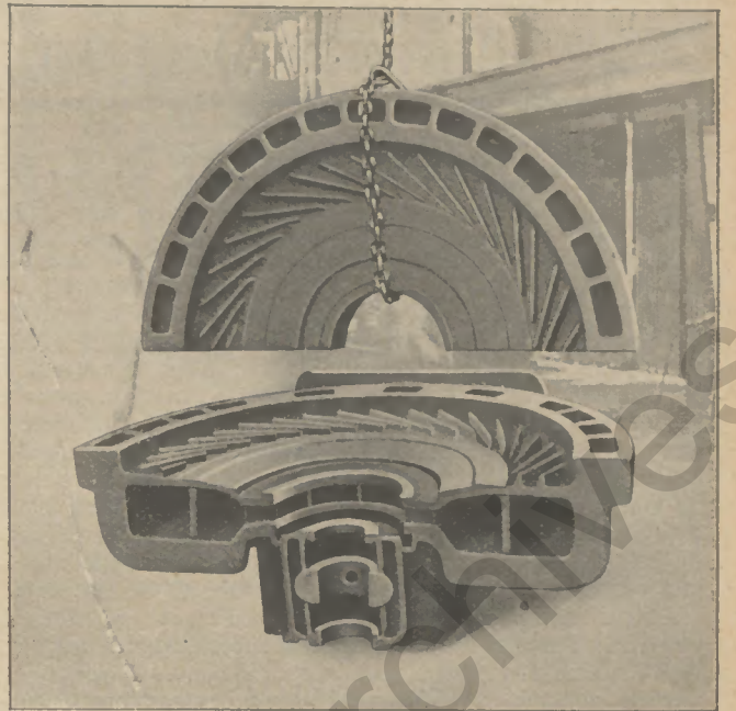
Oben: Saugseitendeckel aus Grauguß für Kompressoren
