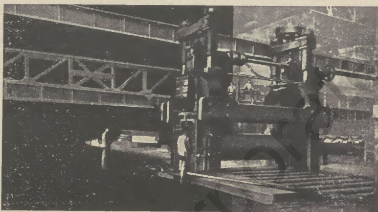
Umkehrwalzenstraße für Grobbleche
