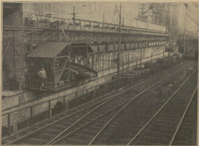
Koks-Bunternanlage mit Koks-Verlade- und Siebwagen.
