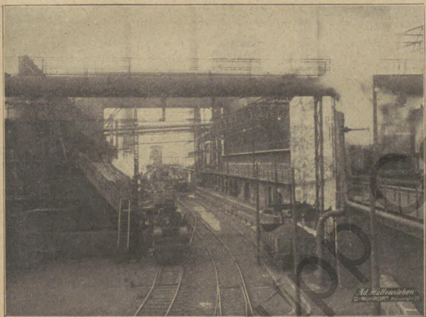
Heutige Kokereianlage.
