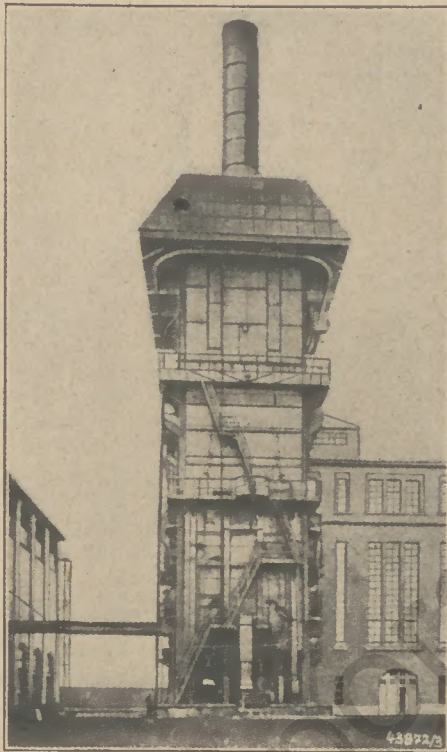
Kohlenstaub-Bensonkessel, maximale Leistung 130 Tonnen pro Stunde, der Centrales Electriques des Flandres et du Brabant, Belgien, gebaut von SSW
