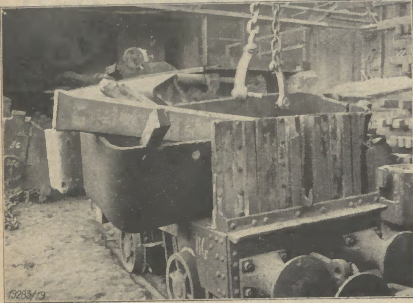
Die rechtwinklige Kopfswand des Wagens reißt den Kettenhaken aus dem Muldenloch heraus
