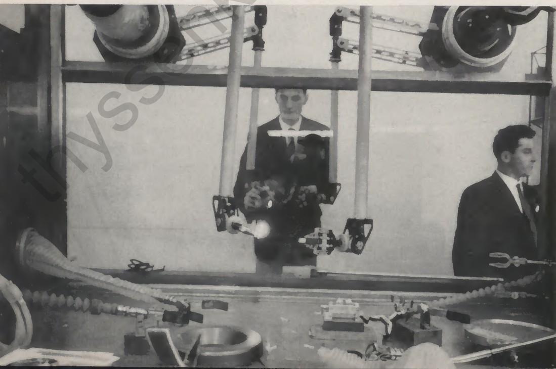
Hände für den Umgang mit radioaktiven Stoffen ▼
