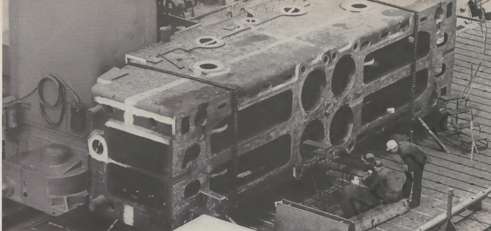
▲ Stahlguß-Kopfstück einer Vierpunkt-Rahmenpresse
