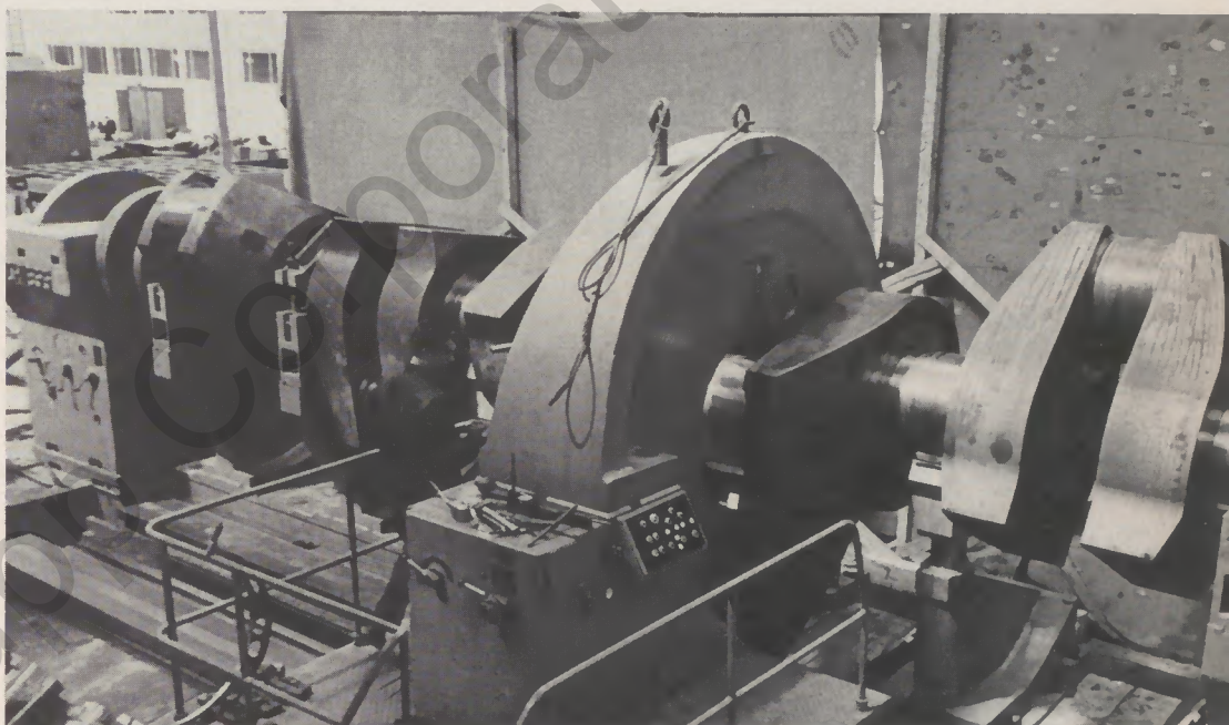
▲ Kurbelwelle auf dem Kurbelzapfen-Drehapparat
