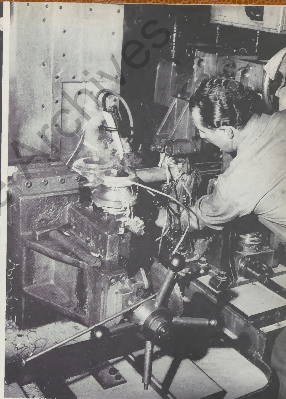
⑦ Schweißaggregat einer Rohrschweißstraße mit Ringspule.
