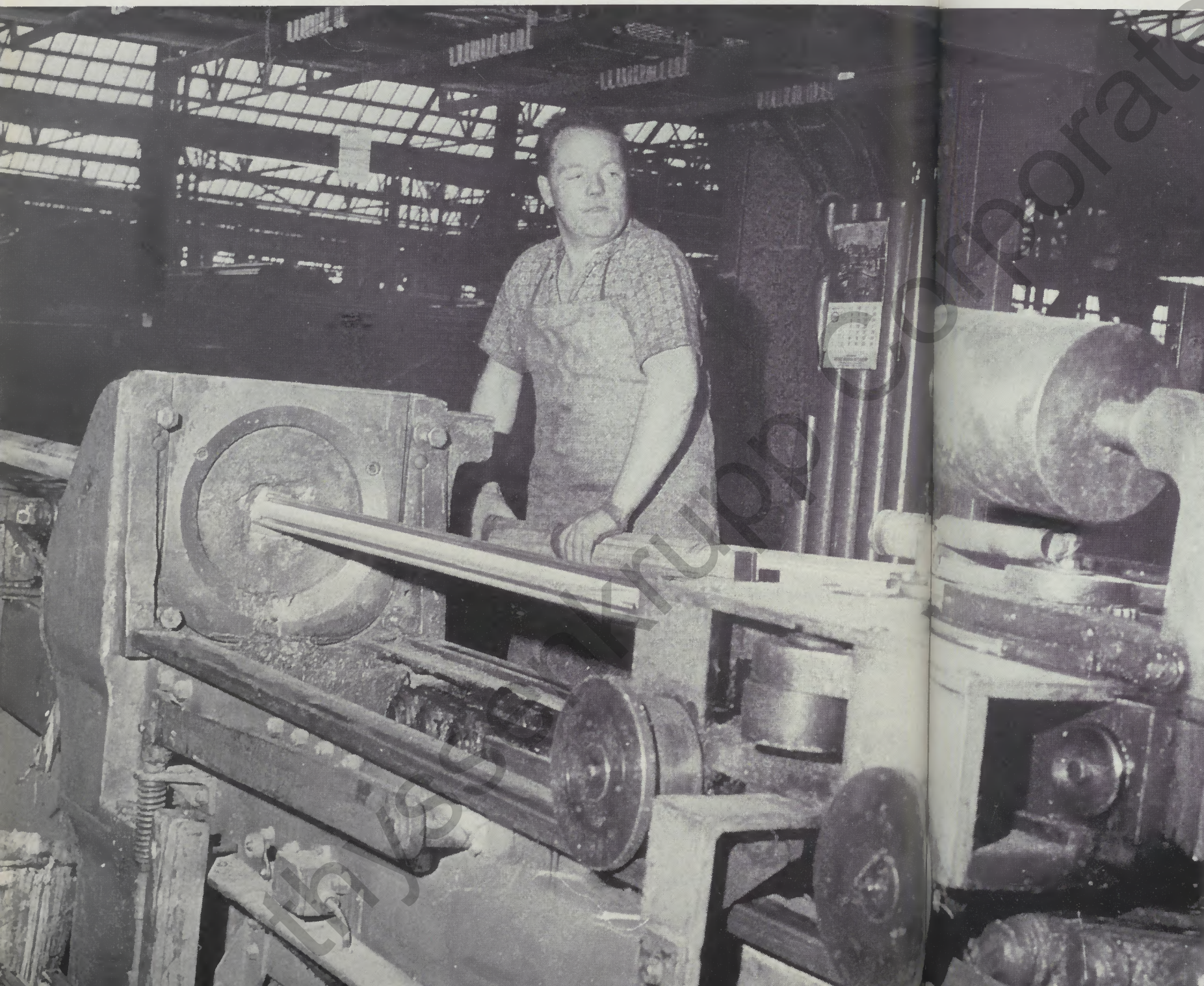
8 Die Kaltziehbank verformt die runden Rohre ...
