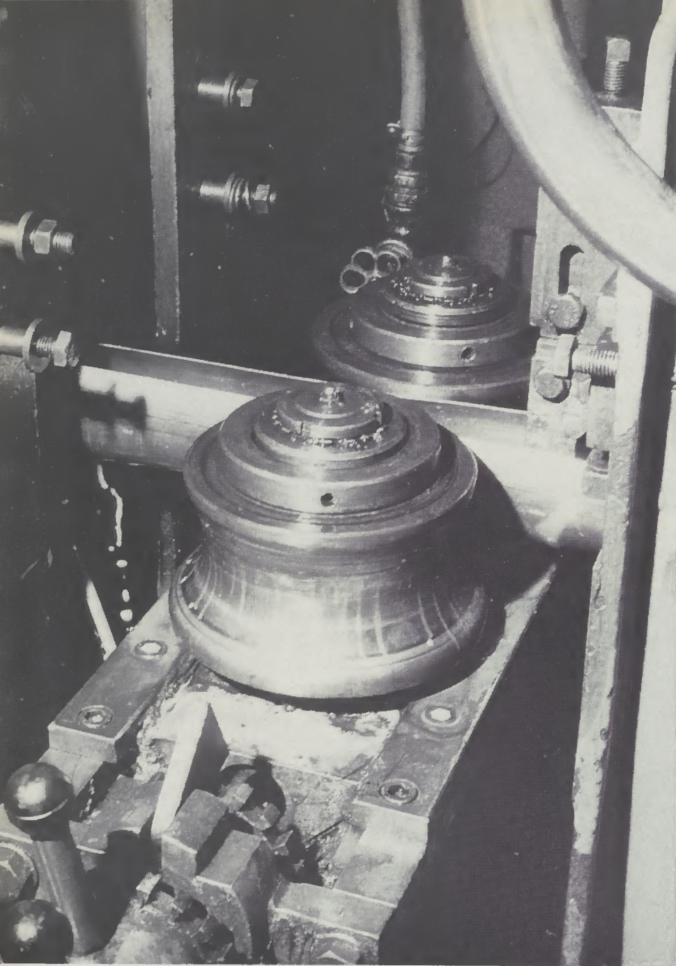
⑤ Von Ständer zu Ständer wird das Band zum Schlitzrohr verformt.
