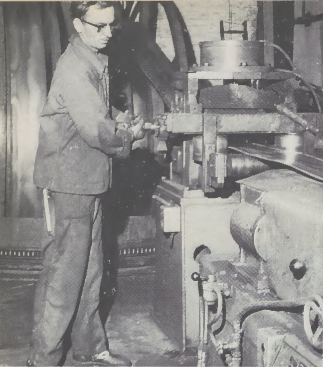
② Auf der Doppeldrehhaspel werden die Bandstahlringe zu einem endlosen Band zusammengeschweißt.
