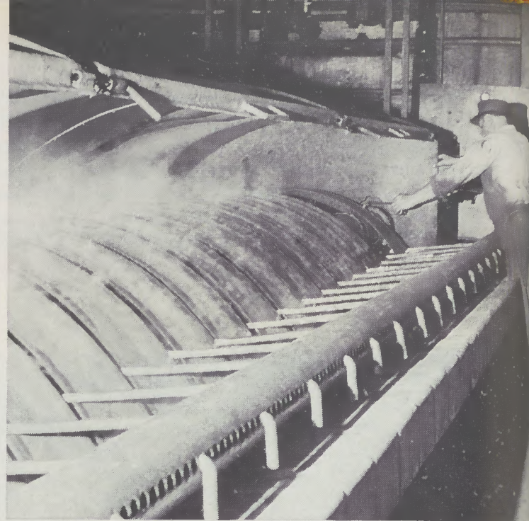
③ Der Bandstahl wird zum Entzundern spiralförmig durch die behelzten mit verdünnter Schwefelsäure gefüllten Beizbecken geführt.
