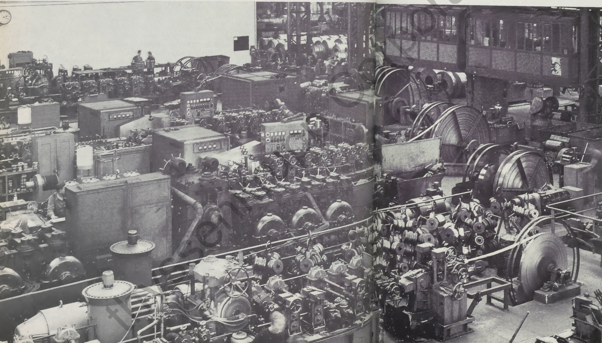
② Auf der Doppeldrehhaspel werden die Bandstahlringe zu einem endlosen Band zusammengeschweißt.
